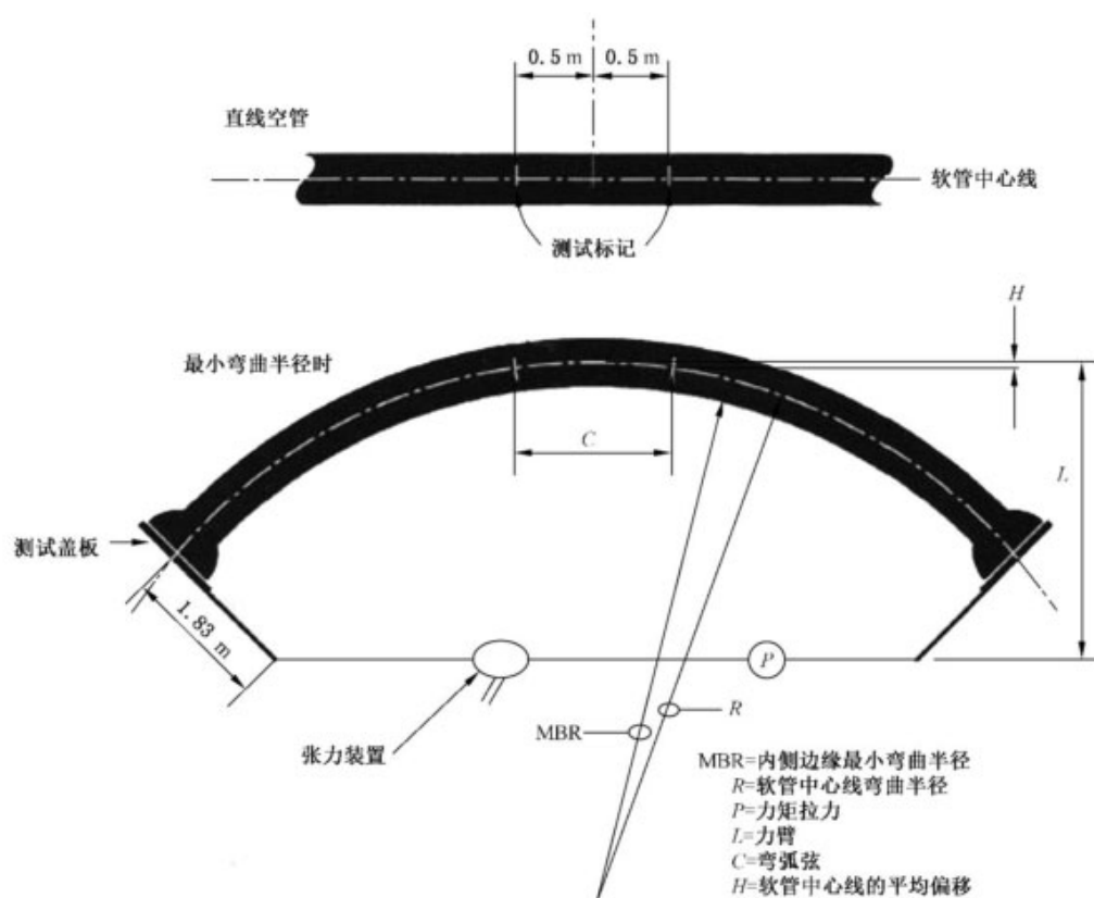
图 D.1 弯曲挺性试验
